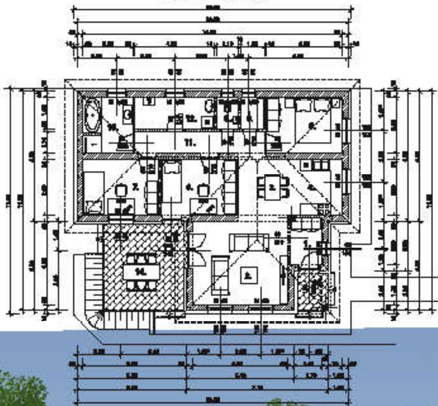
ALAPRAJZ M 1:100
